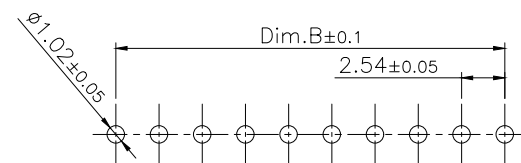
P.C.B Layout
