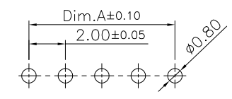
P.C.B Layout
