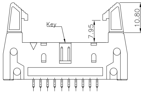
Long Ejector
