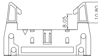
Long Ejector(B Type)
