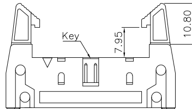
Long Ejector
